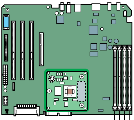
SDRAM DIMM Slots (4)
